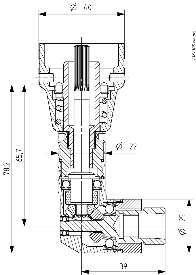
Renvoi d'angle / Angle wrenche CPN 53430641 / PN 381508
